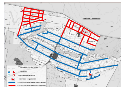
Рисунок 2.4.9.1 - Расположение существующих и перспективных объектов системы водоснабжения с. Верхнее Санчелево.
