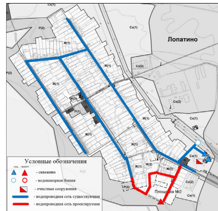
Рисунок 2.4.9.2 - Расположение существующих и перспективных объектов системы водоснабжения с. Лопатино
